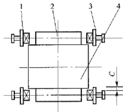
(c) 闸瓦和闸座位置
