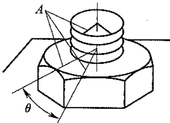
图 5.2.4-2 螺母转角法
