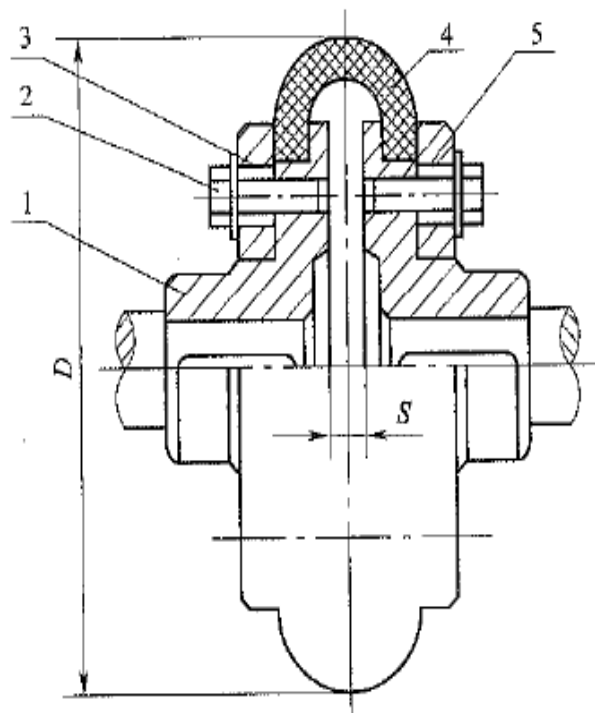
图 5.3.11 轮胎式联轴器
