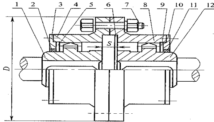
图 5.3.6 齿式联轴器
