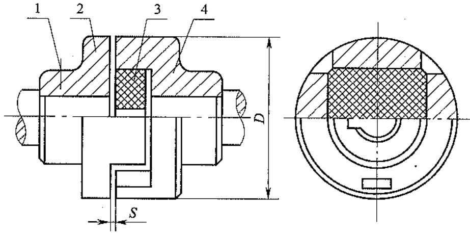
图 5.3.5 滑块联轴器
