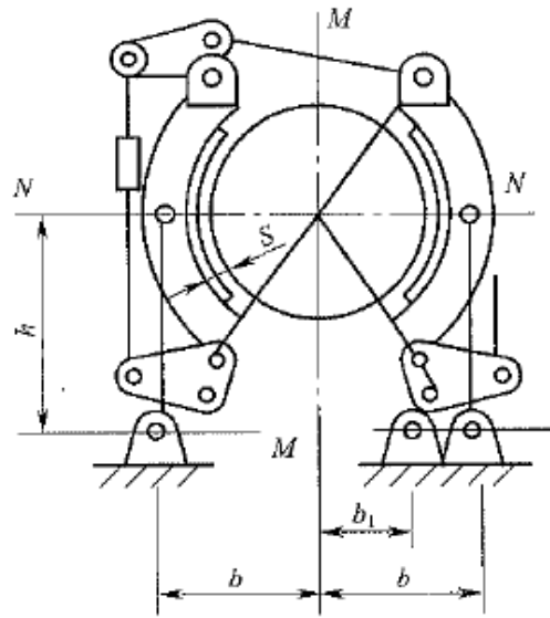
(a) 平移制动器
