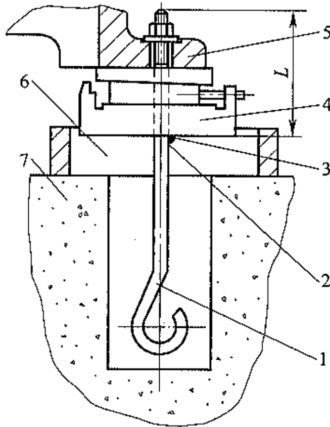
图 C.0.1 压浆法
