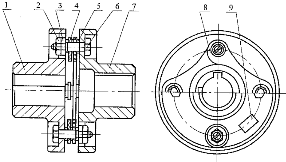
图 5.3.10 膜片联轴器
