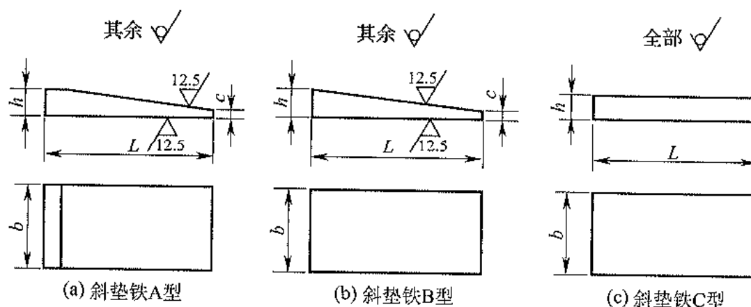
图 A.0.2 斜垫铁和平垫铁
