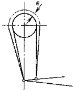
图 5.4.9 带式制动器
