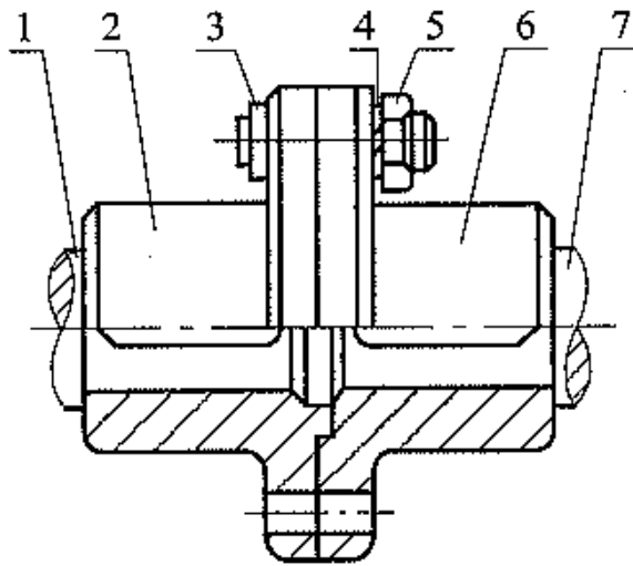
图 5.3.3 凸缘联轴器
