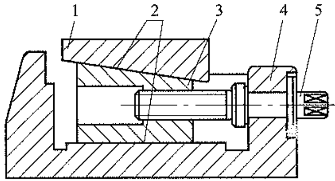
图 4.2.7 螺栓调整垫铁
